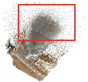
TokenGS-All
