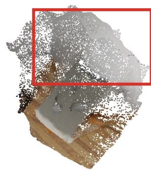
TokenGS-Depth
