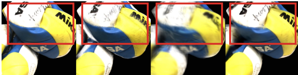
AnySplat*
